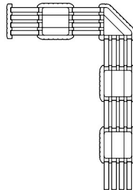
Eckausbildung bis H = 1,50 m
