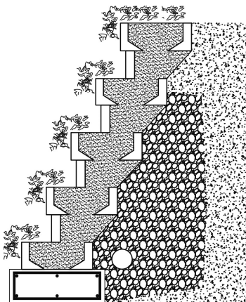
Querschnitt
